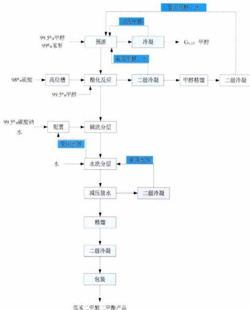
图1 邻苯二甲酸二甲酯生产工艺流程图
