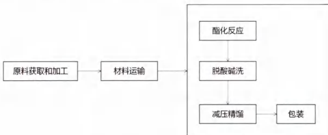
图2 生产1吨邻苯二甲酸二甲酯碳足迹评价系统边界图
